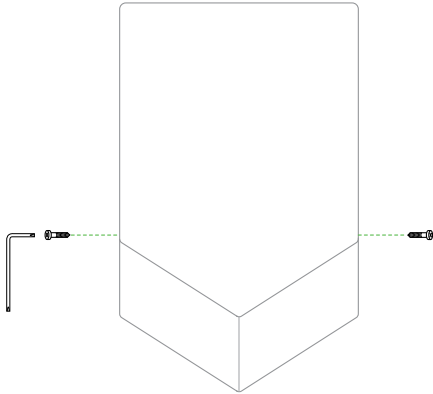
Задна пластина
